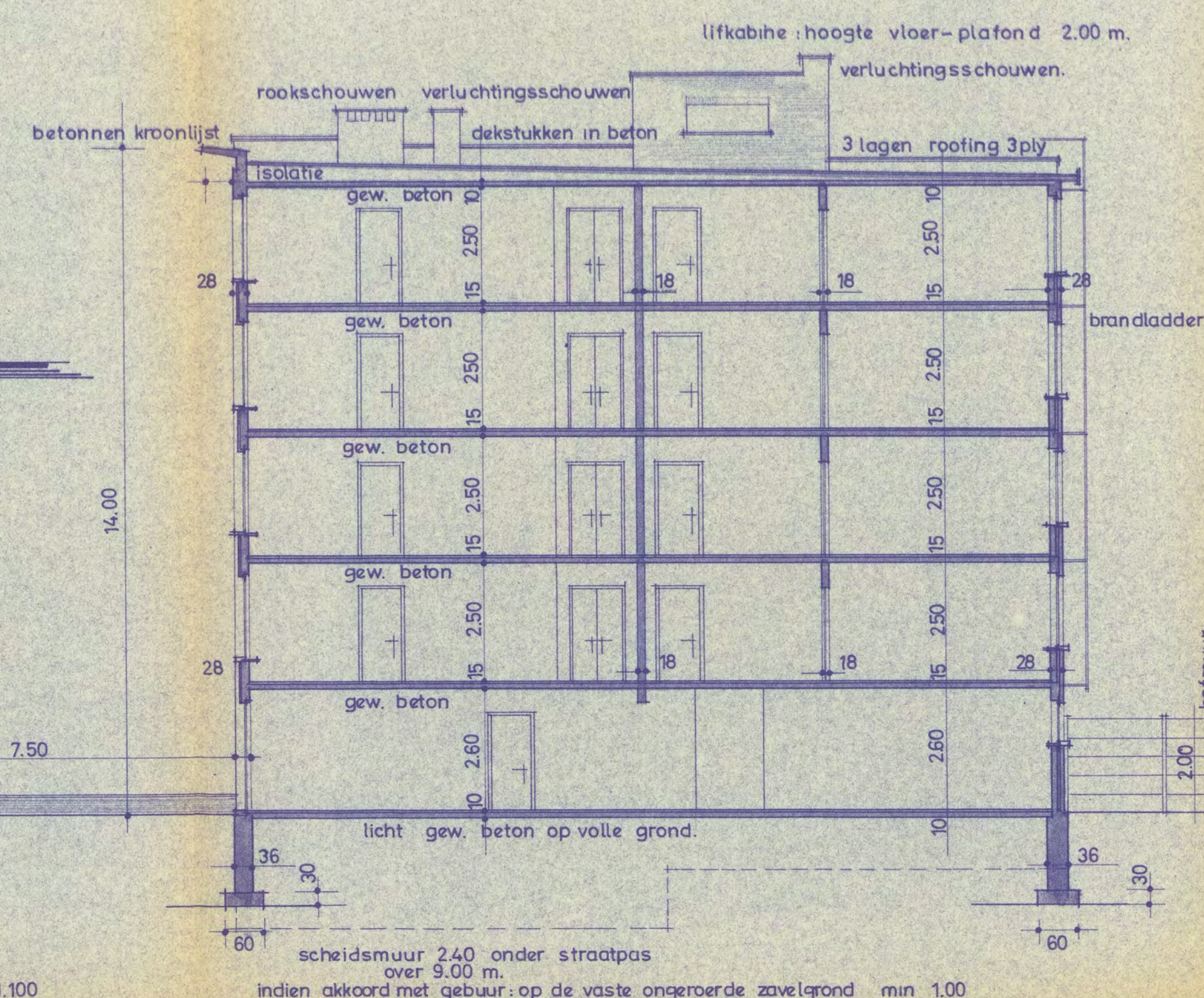
doorsnede a-b.
